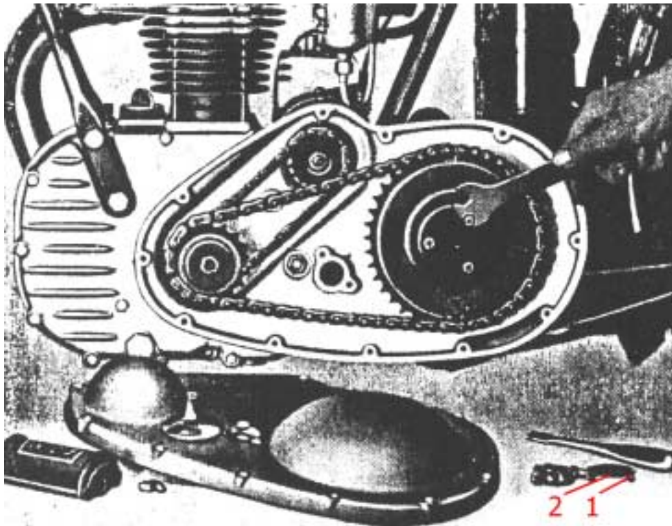
Abb. 3 – Antriebsgehäuse, geöffnet
