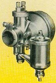
GRAETZIN-Zweikolbenvergaser Type Ke für Bowdenzugregulierung.
