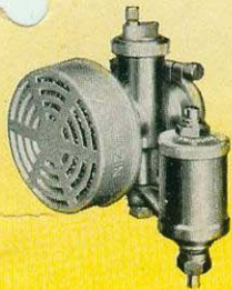
GRAETZIN-Einkolbenvergaser Type Kf für Bowdenzugregulierung.
