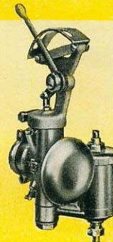
GRAETZIN-Einkolbenvergaser Type Kf für Handregulierung.
