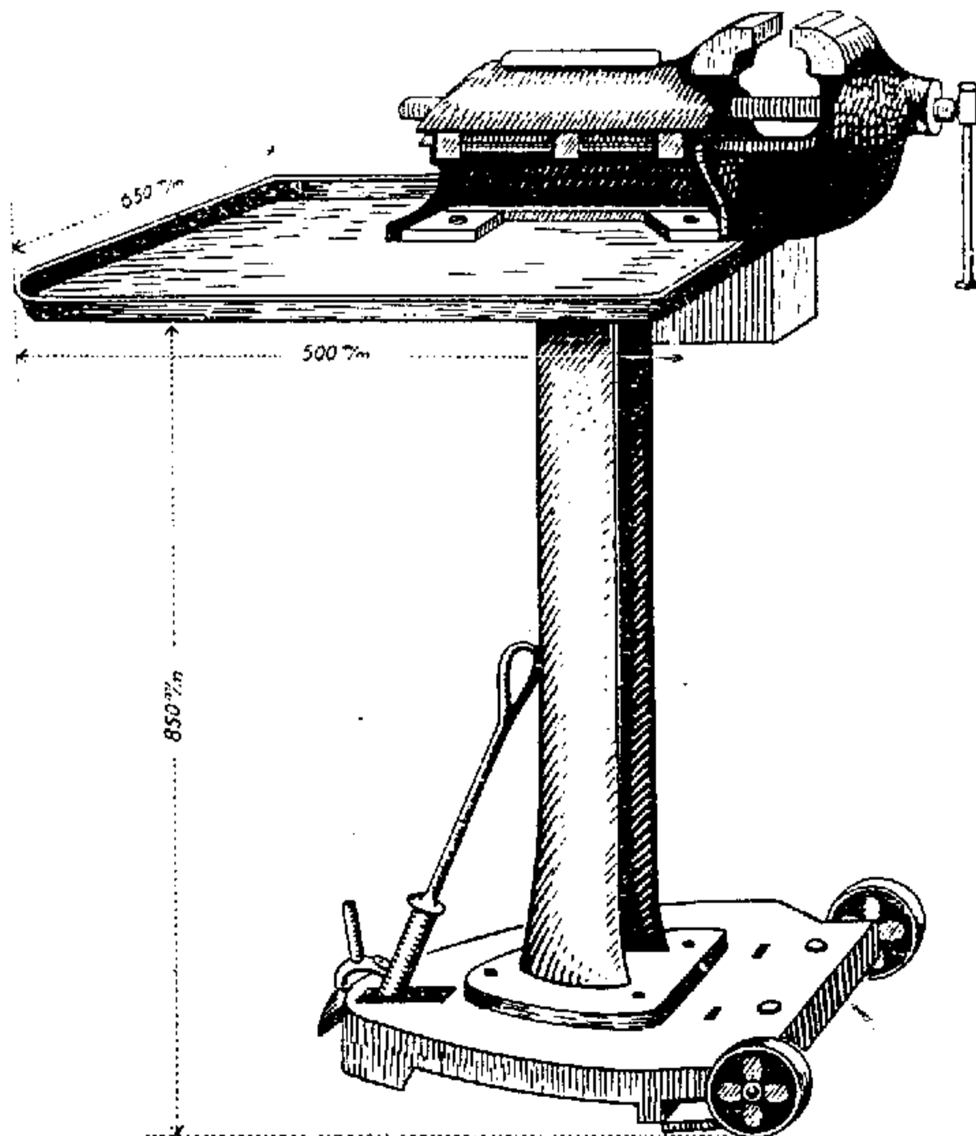
Fahrbarer Montagetisch mit Schraubstock
