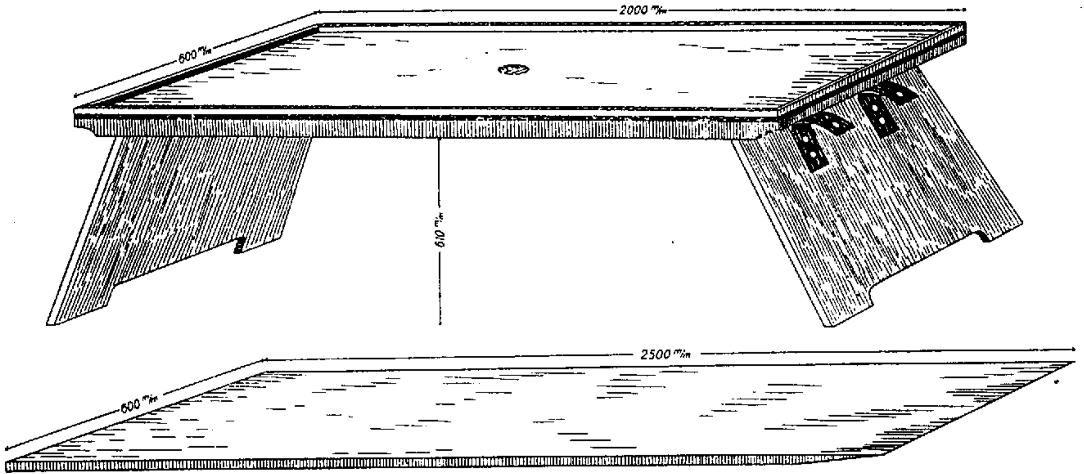
Montagerampe mit Auffahrbrett
